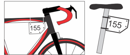
Rahmennummern montieren
